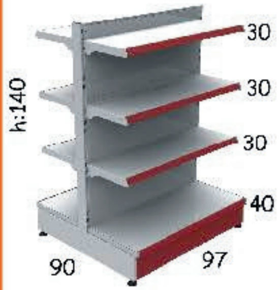
Eko Çiftli Orta Reyon
