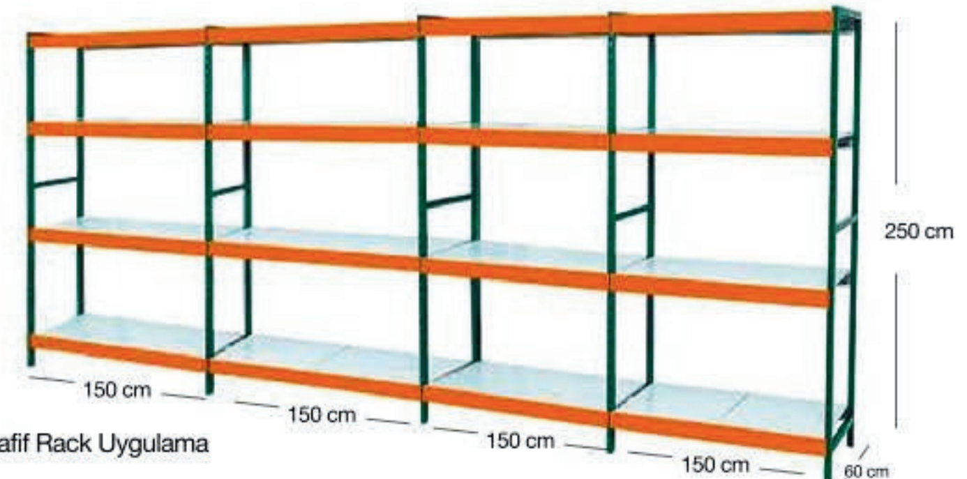
Hafif Rack Uygulama
